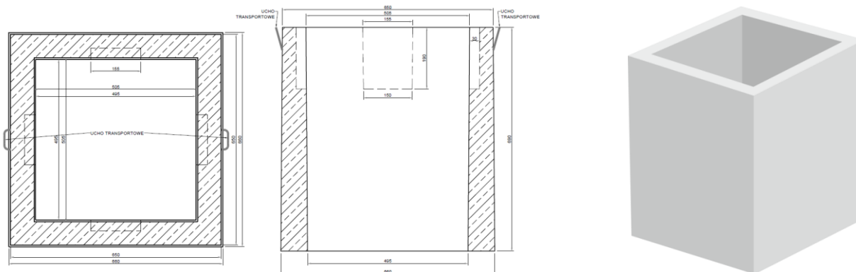
Korpus studni kablowej SK-1(1) D400
