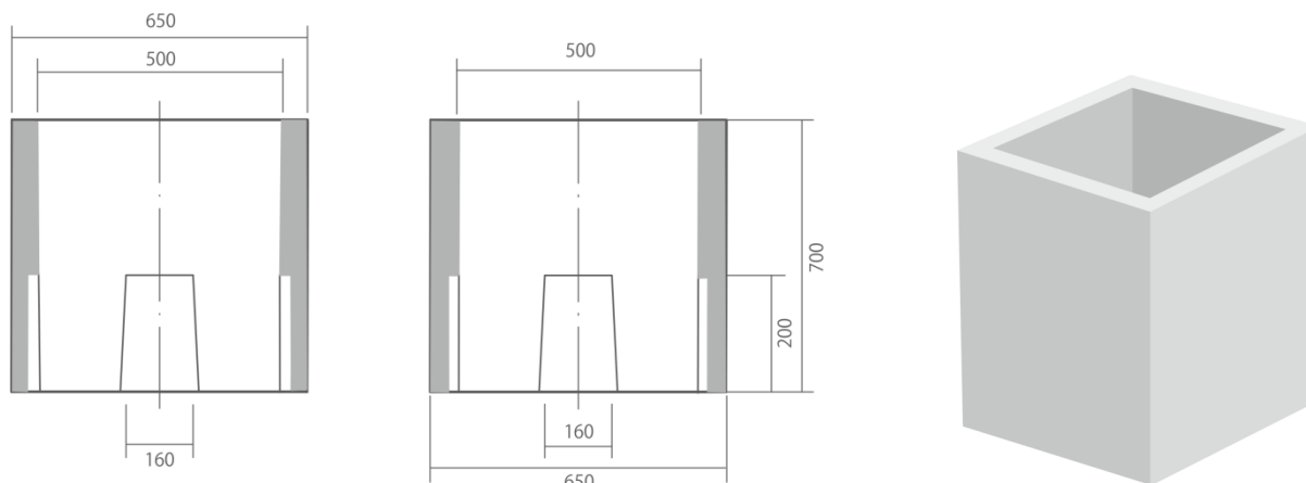
Korpus studni kablowej SK-1(1) A15
