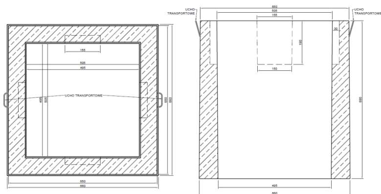
Korpus studni kablowej SK-1(1) C250
